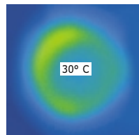
Temperatur der geschliffenen Fläche nach 2 Minuten – mit dem 8-Loch Jetstream-Prinzip.
